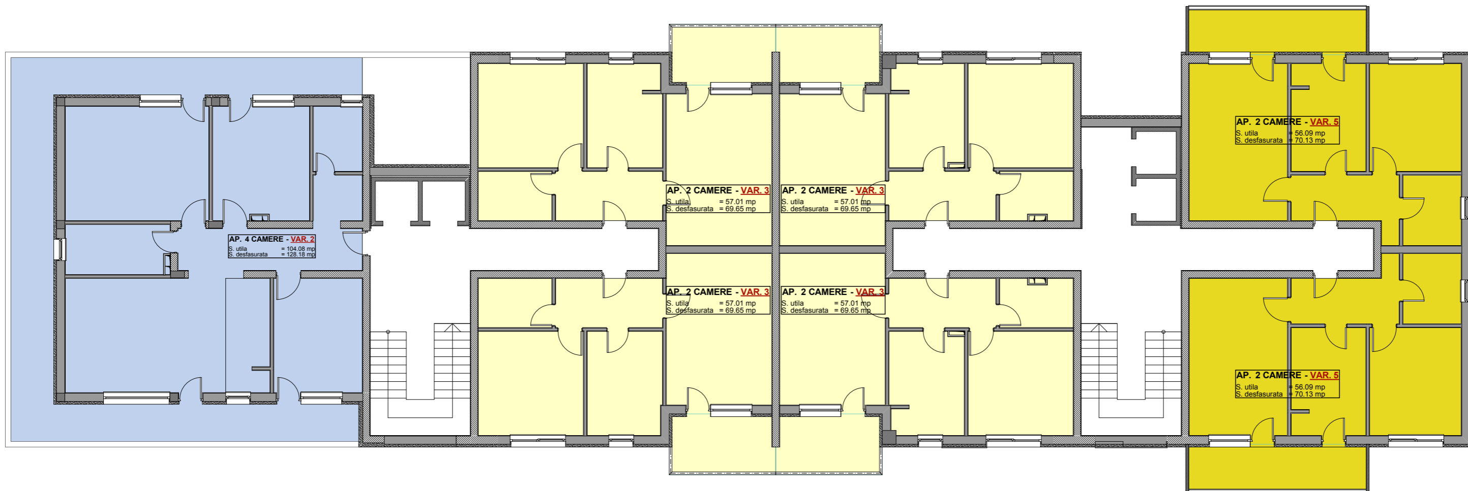
plan etaj 6_et. retras BLOC C
